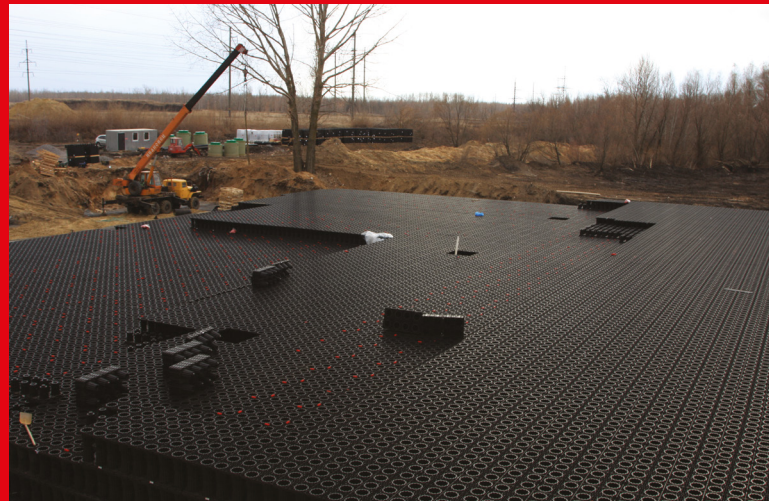
■ Аккумулирующая емкость объемом 6050 м 3 в составе очистных сооружений канализации Индустриального парка "Масловский", г. Воронеж
