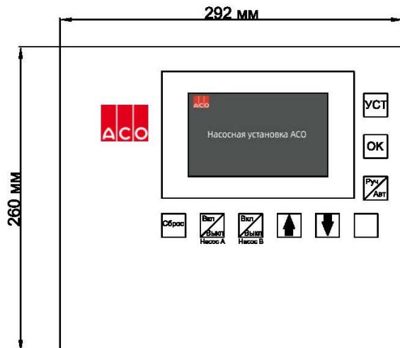
Рисунок 15 – Габаритные размеры шкафа управления
