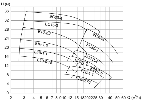
Параметры производительности
