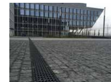
Офисный парк Comcity, Москва Каналы ACO Multiline
